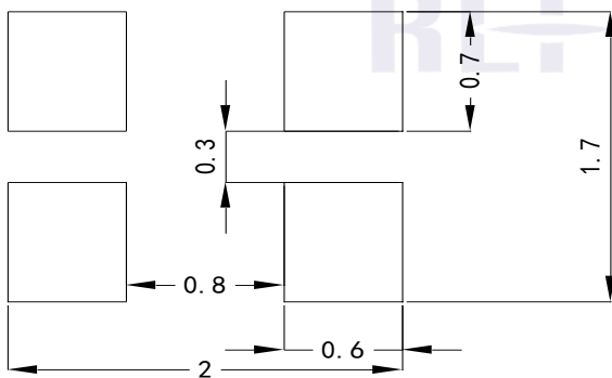
Fig.1-3 Bottom view 背面视图
