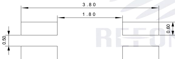
Fig.1-3 Bottom view 背面视图
