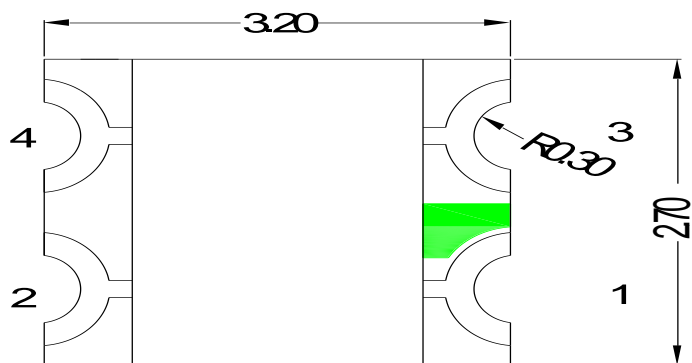
Fig.1-1 Top view 正面视图
