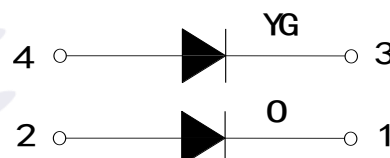
Fig.1-4 Polarity 极性
