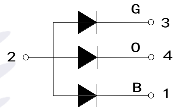
Fig.1-4 Polarity 极性
