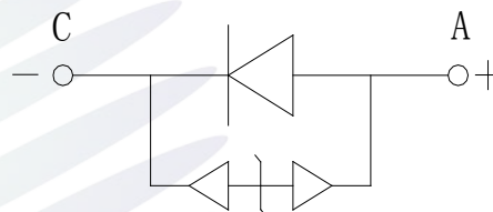
Fig.1-4 Polarity 极性
