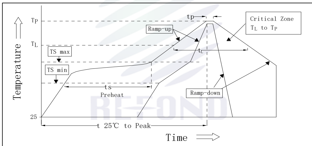
Fig.3-1 Profile 曲线
