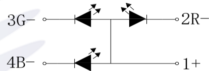
Fig.1-4 Polarity 极性
