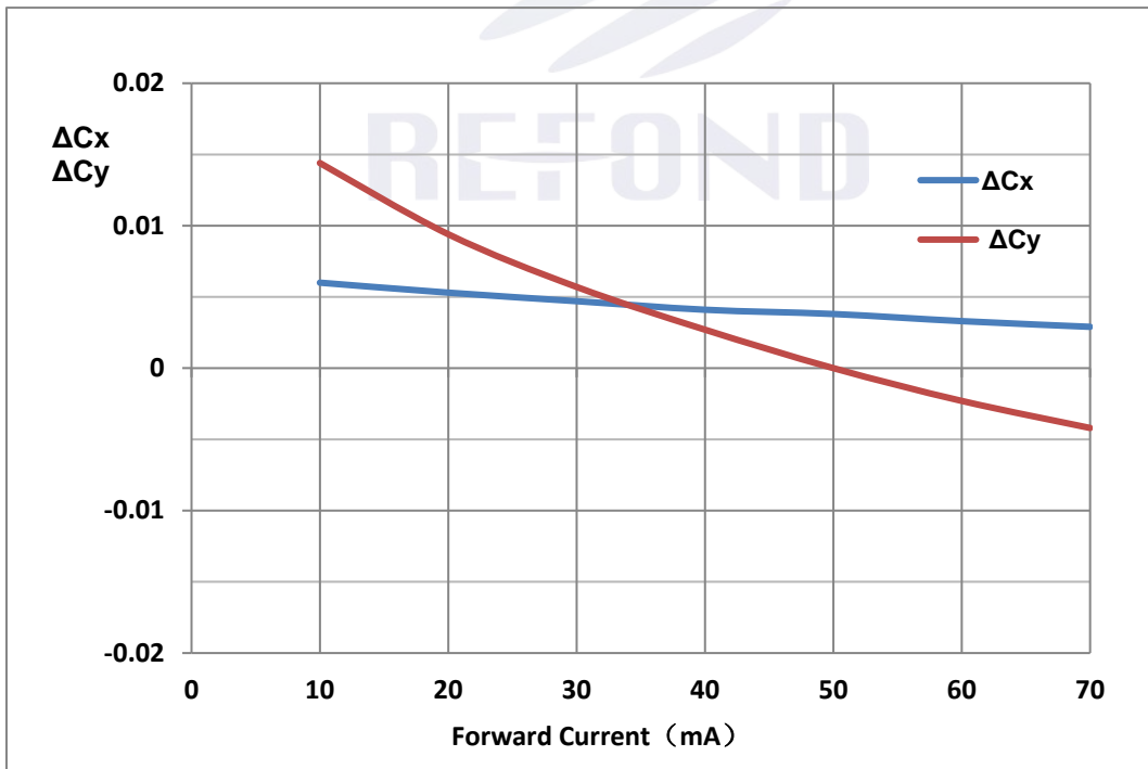
Fig. 1-14 Color coordinate shift Vs Forward Current 色坐标偏移与正向电流特性曲线
