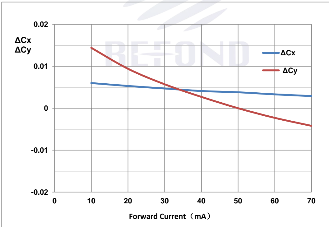
Fig. 1-14 Color coordinate shiftVs Forward Current色坐标偏移与正向电流特性曲线
