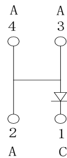
Fig. 1-4 Polarity极性
