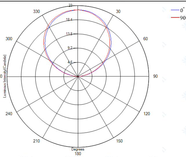
图 10 配光曲线
