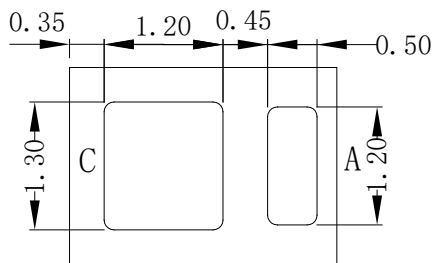
Fig.1-3 Bottom View 背面视图
