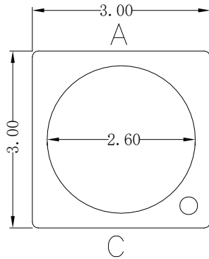
Fig.1-1 Top View 正面视图
