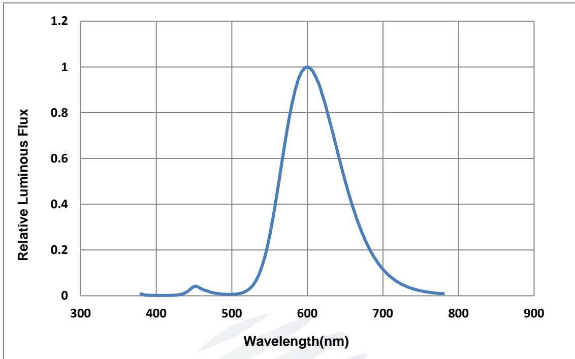
Fig 1-15 Spectrum Distribution 光谱分布特性曲线
