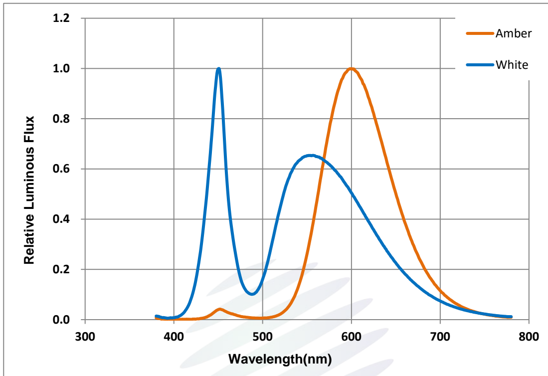
Fig. 1-16 Spectrum Distribution光谱分布特性曲线
