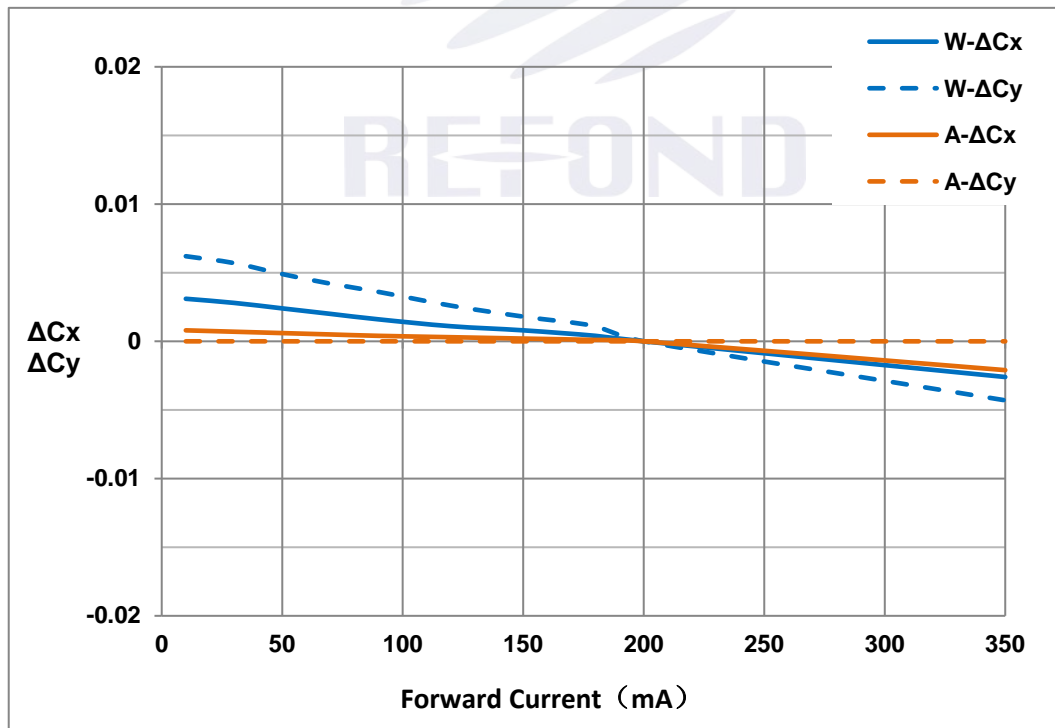
Fig. 1-15 Chromaticity Coordinate Shift Vs Forward Current 色坐标偏移与正向电流特性曲线
